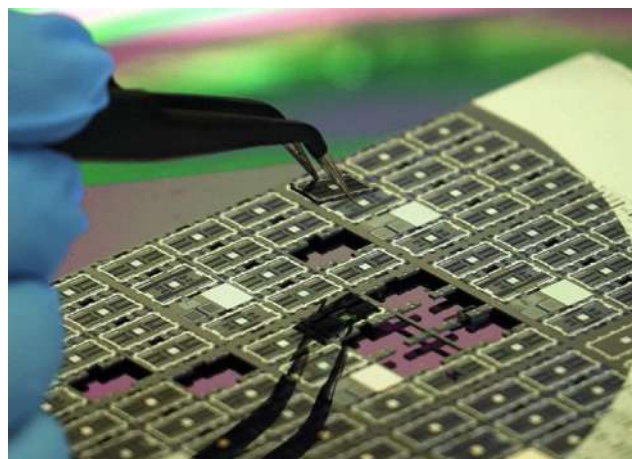
Assemblagem de dispositivos (INL) Assembly of devices (INL)
